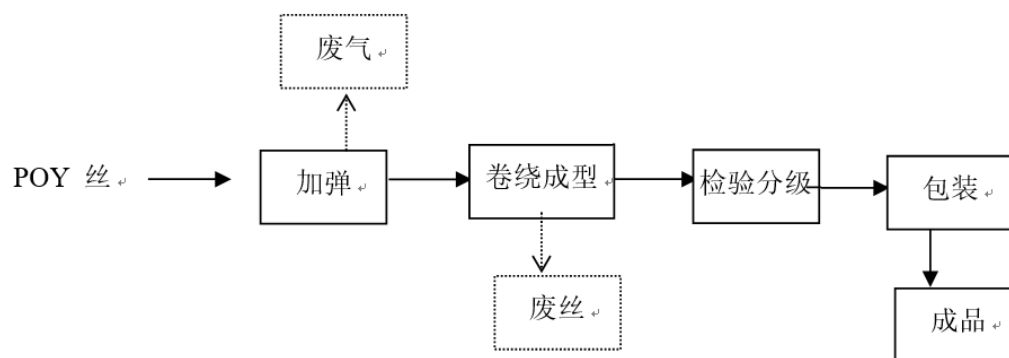
图 2-1 本项目生产工艺流程及产污点位图
