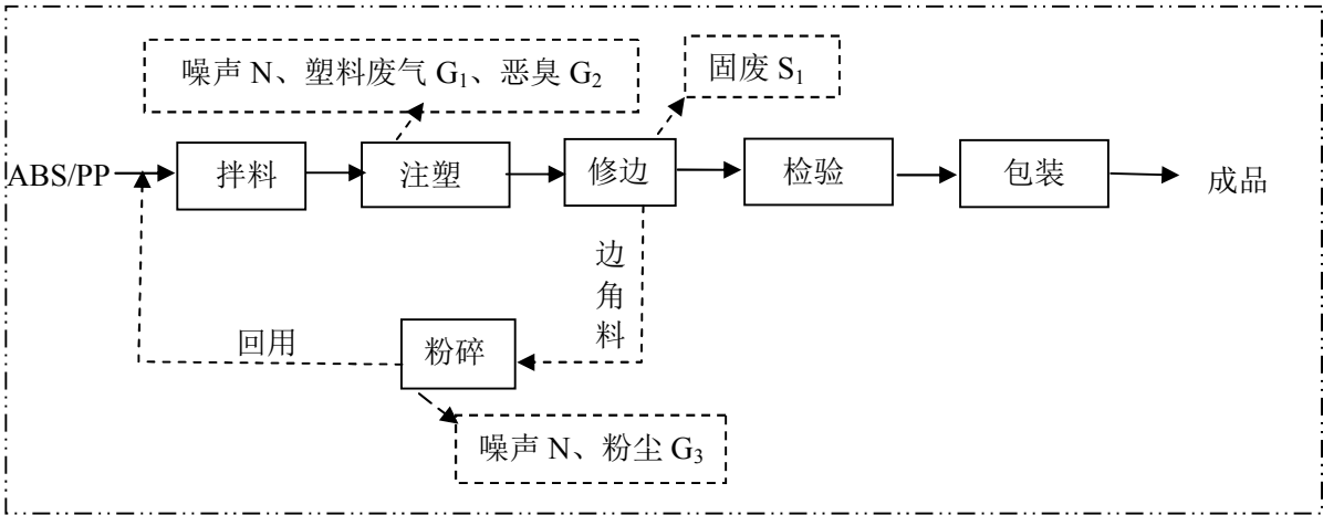
图 5-1 塑料件半成品生产工艺流程和产污环节图
