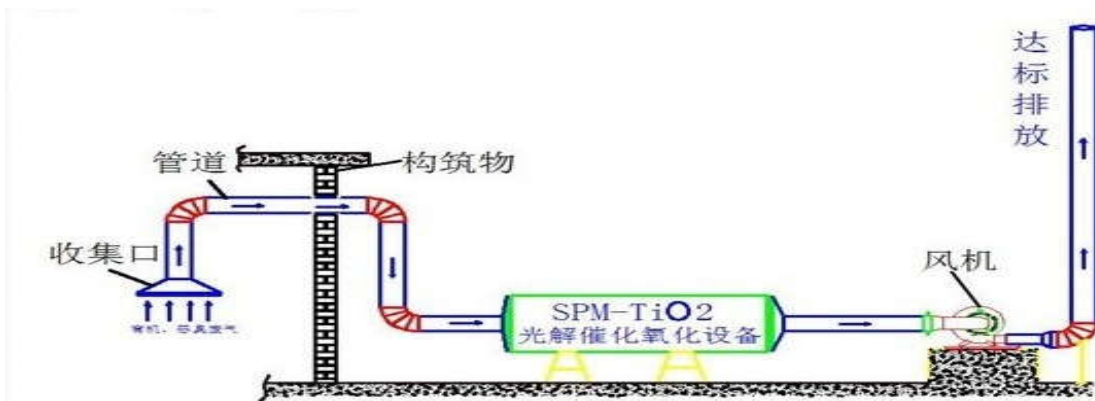
图 8-1 工艺示意图
