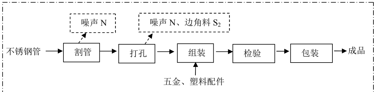
图 5-2 产品生产工艺流程和产污环节图
